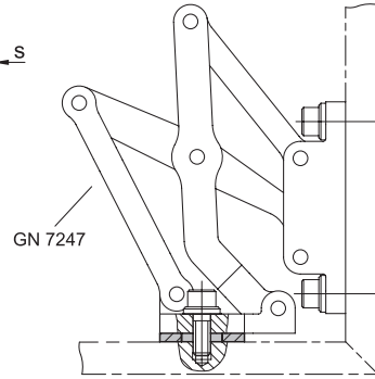
Montaj örneği
